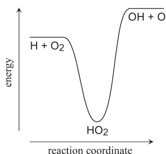
図2 反応 \text{H} + \text{O}_2 \rightarrow (\text{HO}_2) \rightarrow \text{OH} + \text{O} のエネルギーダイアグラム.
